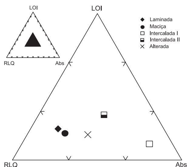
FIGURA 4. Diagrama ternário \text{SiO}_2 - \text{Al}_2\text{O}_3 - \text{Na}_2\text{O}+\text{K}_2\text{O}+\text{CaO}+\text{MgO} para as litofácies cerâmicas (médias das amostras ensaiadas).
