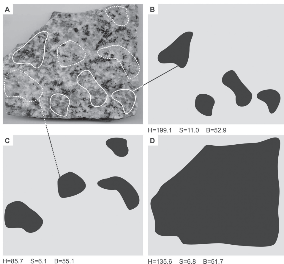
FIGURA 4. Filtros de seleção para análises de cor em rocha total e em spot confeccionados para uma variedade do Granito Azul Bahia: (A) Imagem da rocha. (B) Filtro de seleção para áreas concentradas em sodalita de cor azul. (C) Filtro para áreas concentradas em nefelina de cor cinza. (D) Filtro para análise de cor em rocha total.
