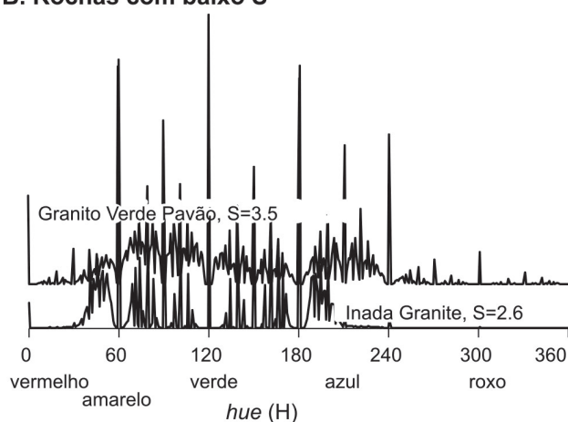
FIGURA 6. Histograma do parâmetro H para rochas ornamentais que têm: (A) alto valor do parâmetro S, Granito Amarelo Icaraí, Granito Azul Bahia e Granito Bege Bahia; (B) baixo S, Granito Verde Pavão e Inada Granite.
